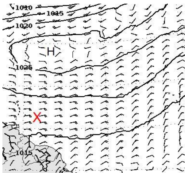
Vorhersage für Freitag 12 UTC
