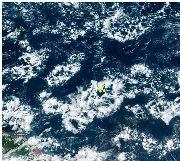
Satellitenbild GOES16 13.02.2020 12:50 UTC
