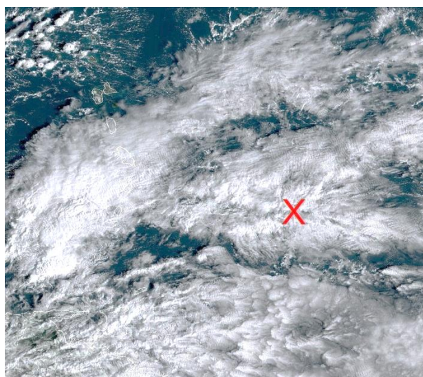
Satellitenbild GOES16 14.02.2020 12:50 UTC
