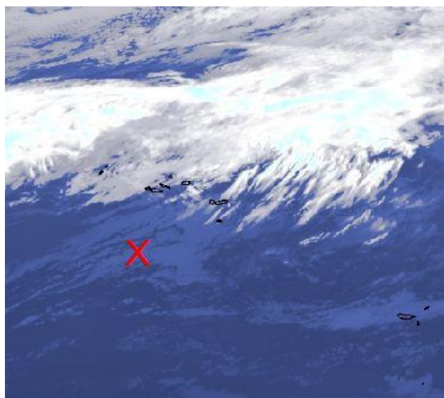
Satellitenbild 01.03.2020 10:00 UTC
