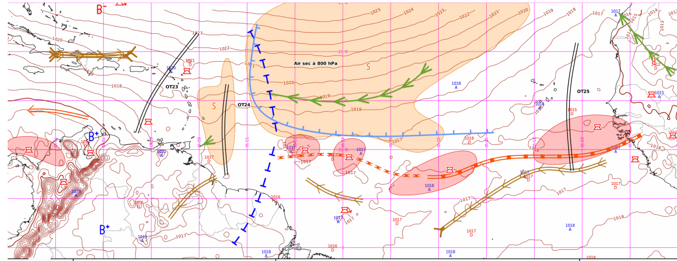
ANASYG du mer. 24/07/2024 - 12 UTC
