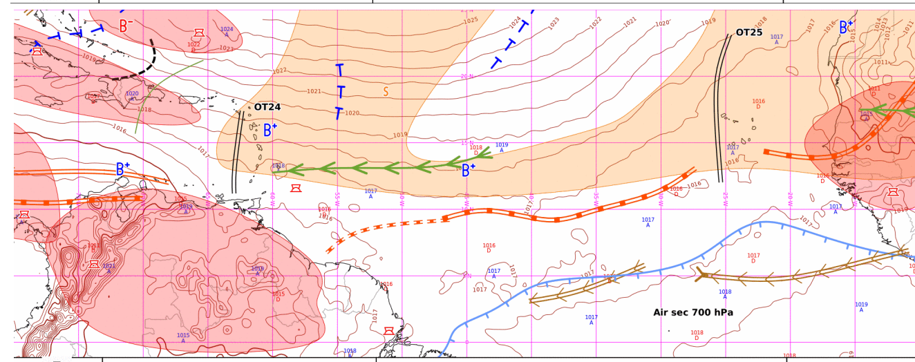
ANASYG du jeu. 25/07/2024 - 00 UTC
