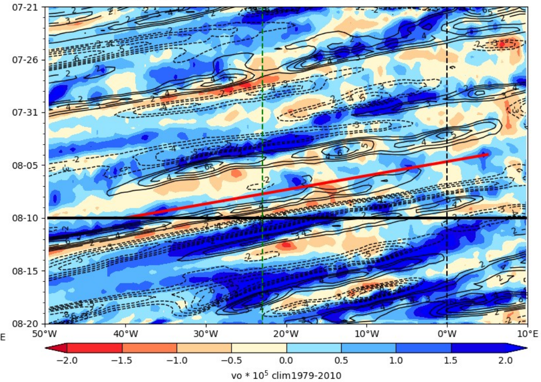
ECMWF Vorticity 850 hPa (color), V-700 hPa 2024-08-10
