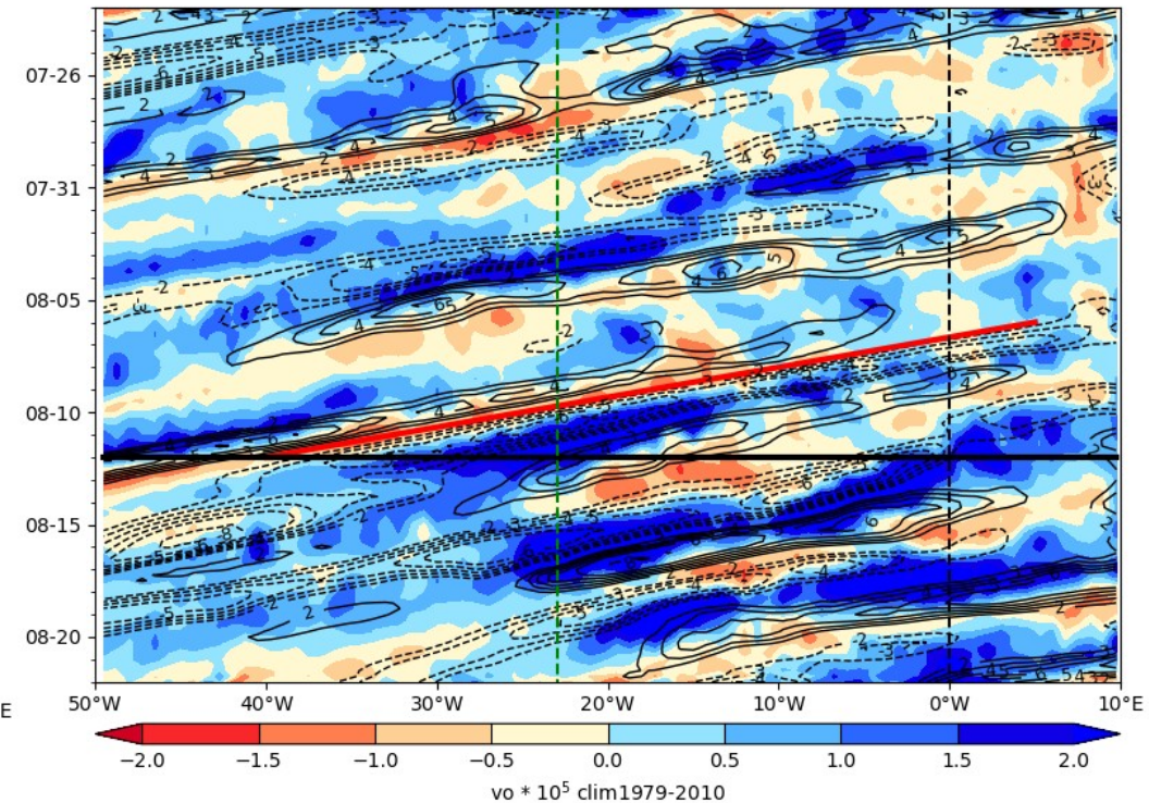
ECMWF Vorticity 850 hPa (color), V-700 hPa 2024-08-12
