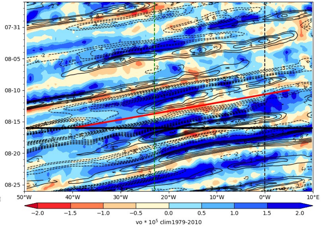
ECMWF Vorticity 850 hPa (color), V-700 hPa 2024-08-16
