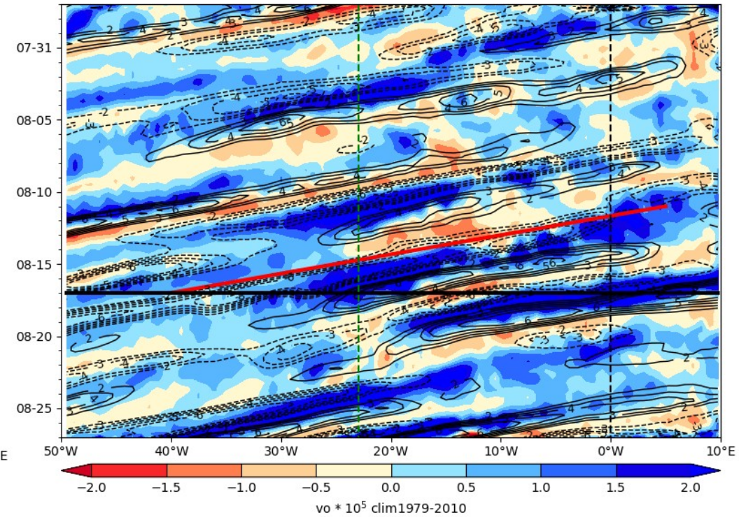
ECMWF Vorticity 850 hPa (color), V-700 hPa 2024-08-17
