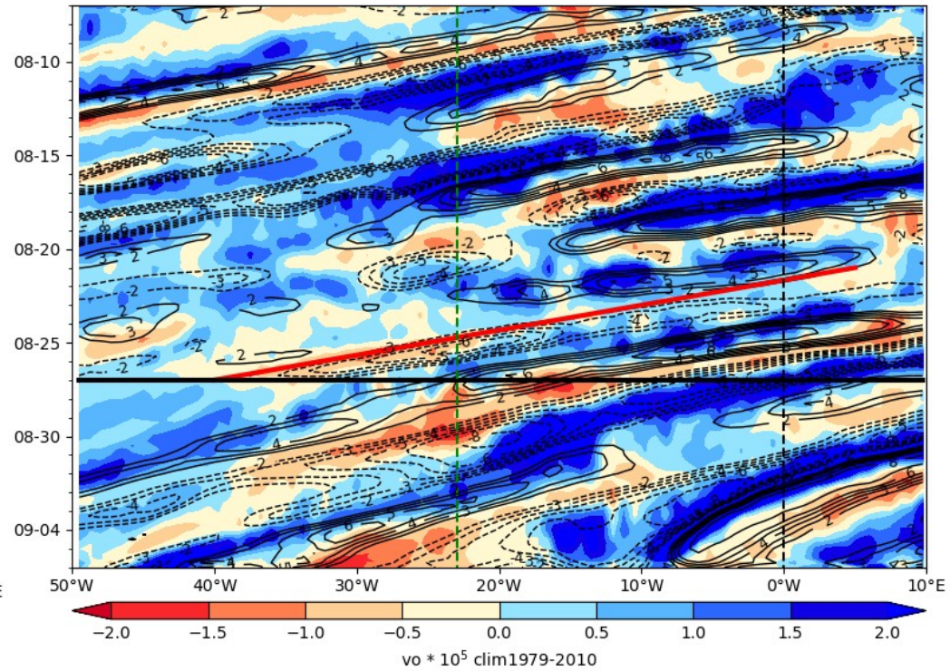
ECMWF Vorticity 850 hPa (color), V-700 hPa 2024-08-27
