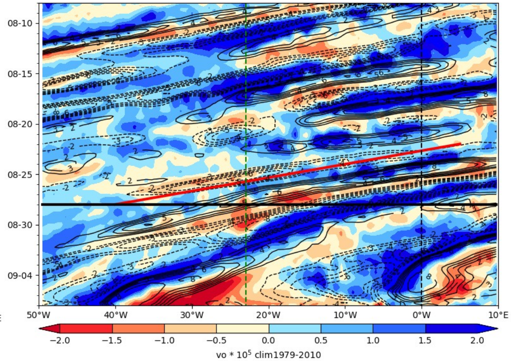
ECMWF Vorticity 850 hPa (color), V-700 hPa 2024-08-28
