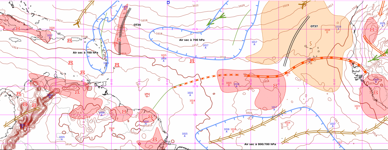
ANASYG du mer. 28/08/2024 - 00 UTC
