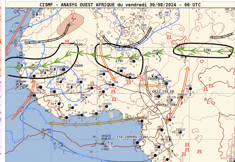
CISMF - ANASYG OUEST AFRIQUE du vendredi 30/08/2024 - 06 UTC
