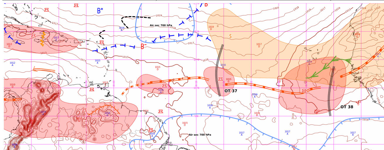
ANASYG du ven. 30/08/2024 - 00 UTC
