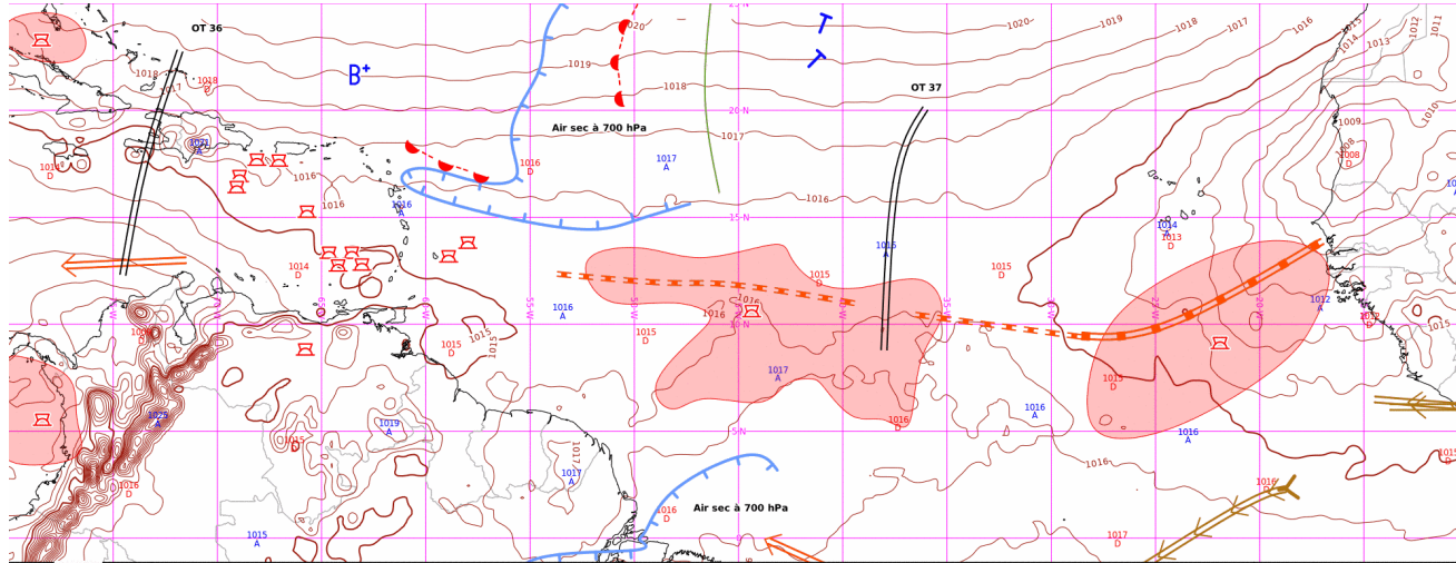
ANASYG du jeu. 29/08/2024 - 12 UTC
