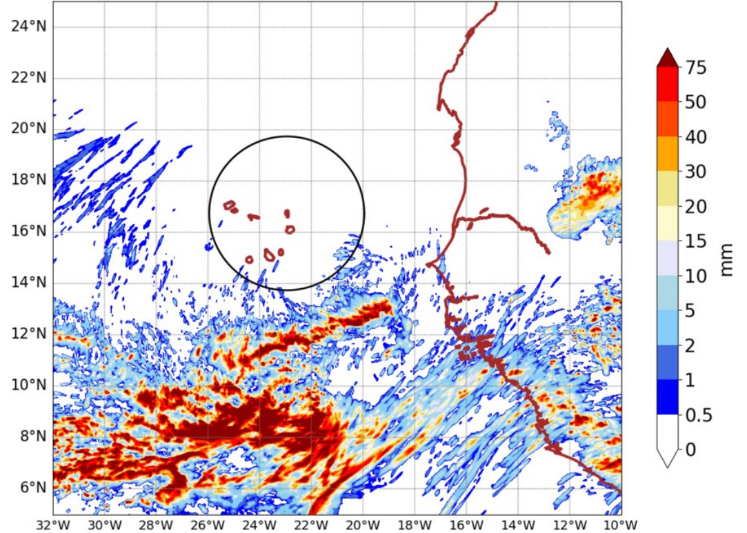
AROME25 20240831-00-UTC -ech(24h)
