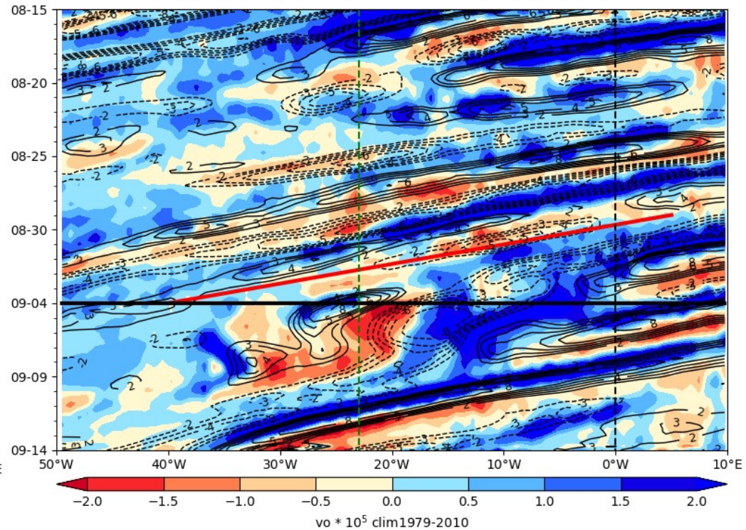
ECMWF Vorticity 850 hPa (color), V-700 hPa 2024-09-04
