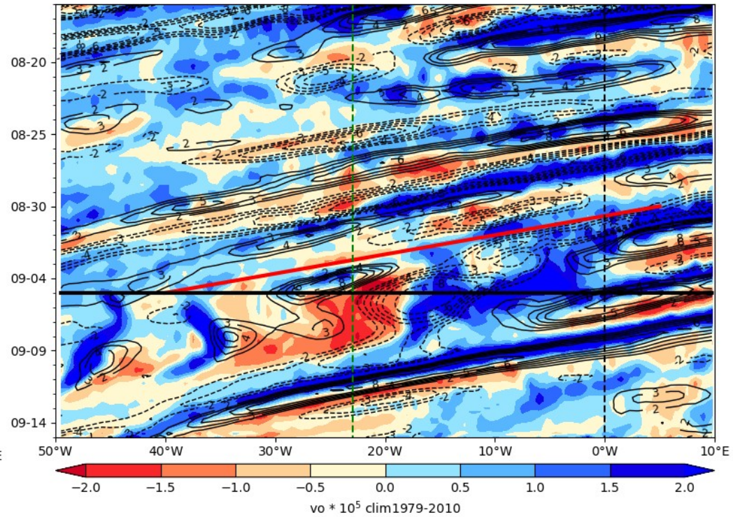
ECMWF Vorticity 850 hPa (color), V-700 hPa 2024-09-05
