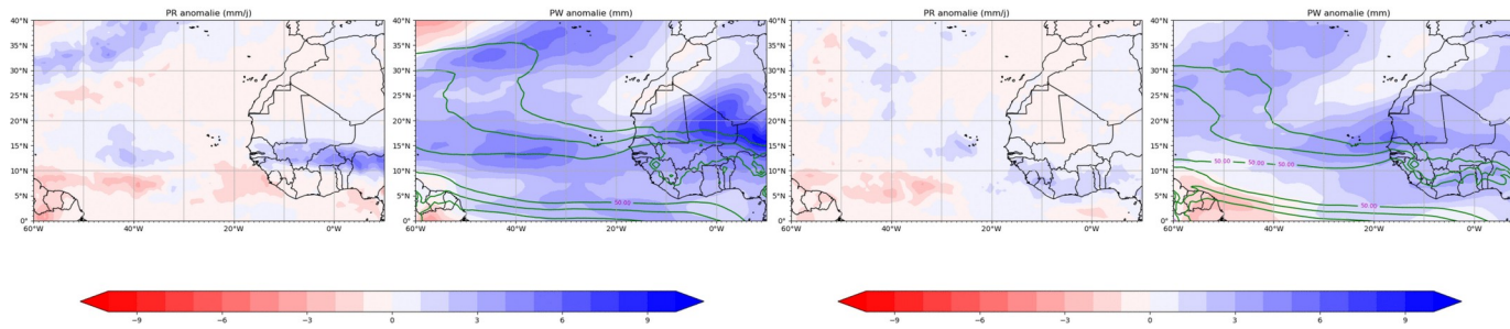
ECMWF EPS Moyenne hebdomadaire PR et PW Anomalie
