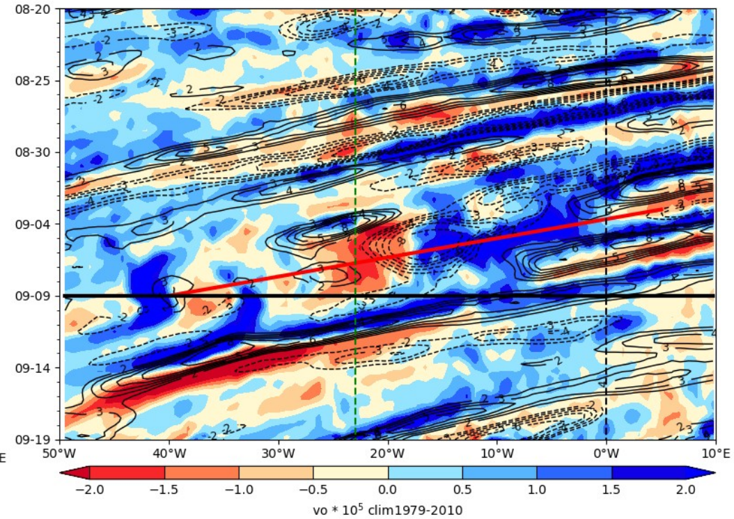
ECMWF Vorticity 850 hPa (color), V-700 hPa 2024-09-09
