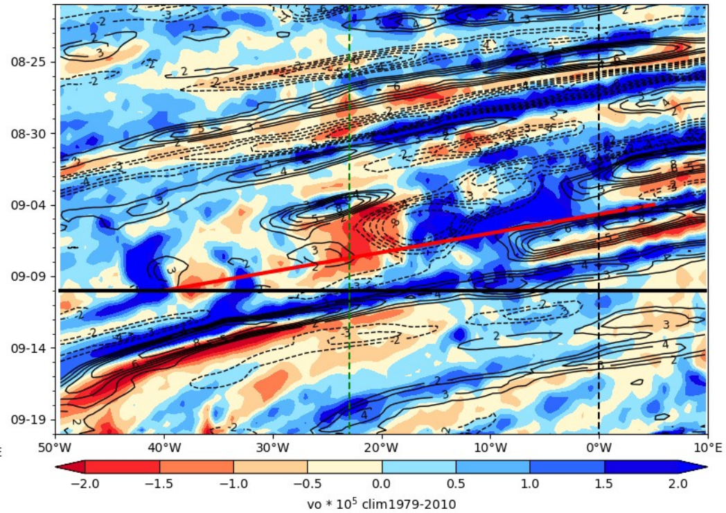
ECMWF Vorticity 850 hPa (color), V-700 hPa 2024-09-10
