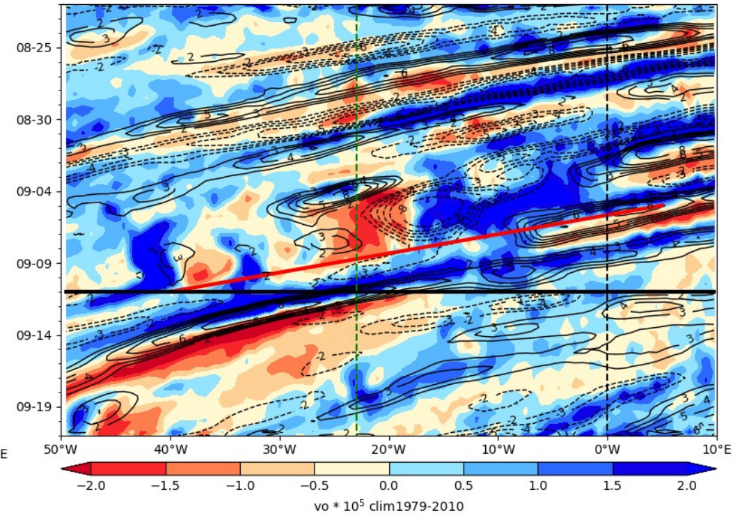
ECMWF Vorticity 850 hPa (color), V-700 hPa 2024-09-11
