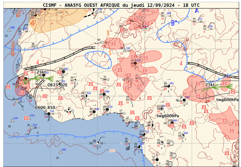
CISMF - ANASYG OUEST AFRIQUE du jeudi 12/09/2024 - 18 UTC
