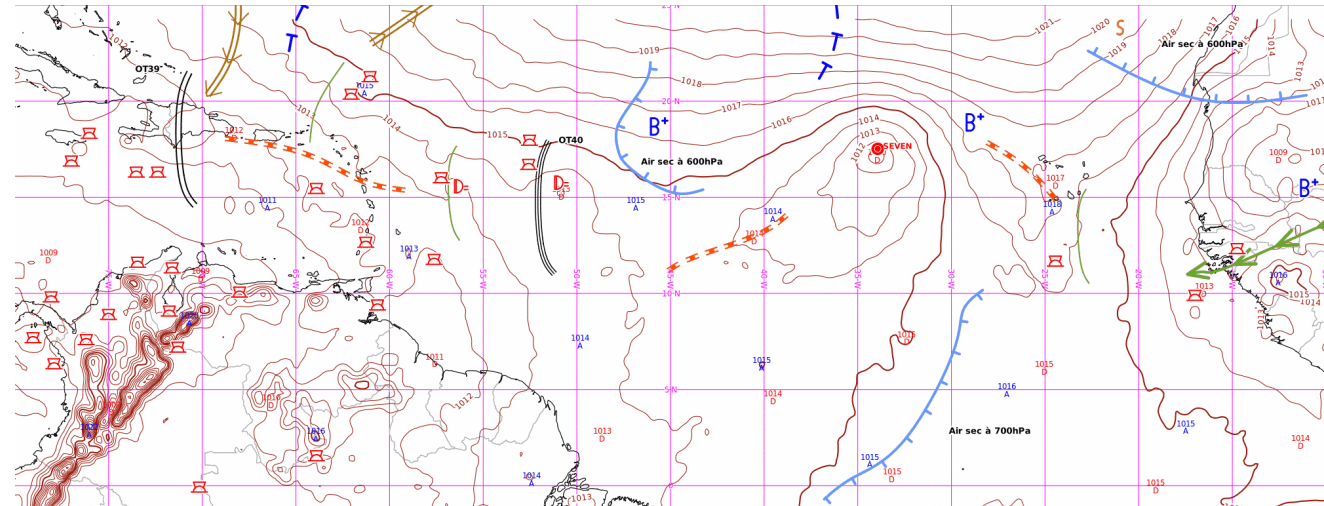
ANASYG du jeu. 12/09/2024 - 12 UTC
