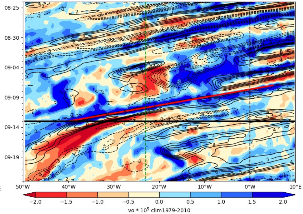
ECMWF Vorticity 850 hPa (color), V-700 hPa 2024-09-13
