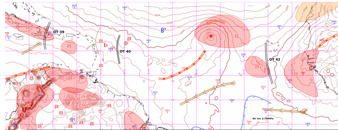
ANASYG du ven. 13/09/2024 - 00 UTC
