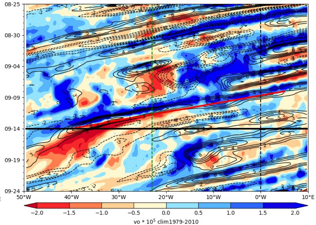
ECMWF Vorticity 850 hPa (color), V-700 hPa 2024-09-14
