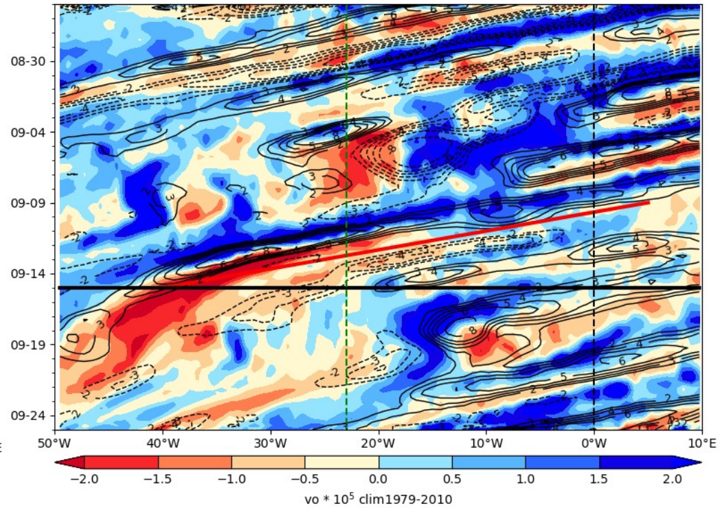
ECMWF Vorticity 850 hPa (color), V-700 hPa 2024-09-15
