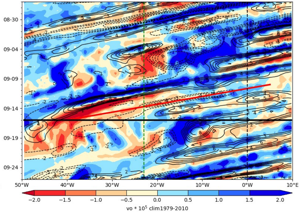
ECMWF Vorticity 850 hPa (color), V-700 hPa 2024-09-16
