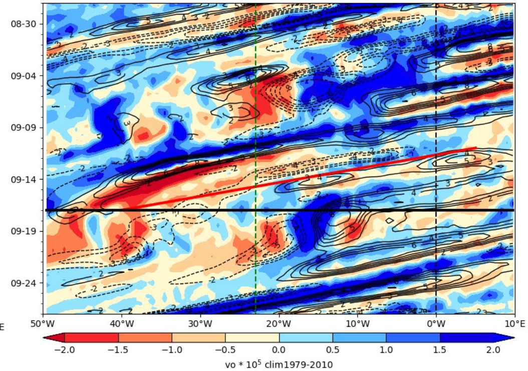
ECMWF Vorticity 850 hPa (color), V-700 hPa 2024-09-17
