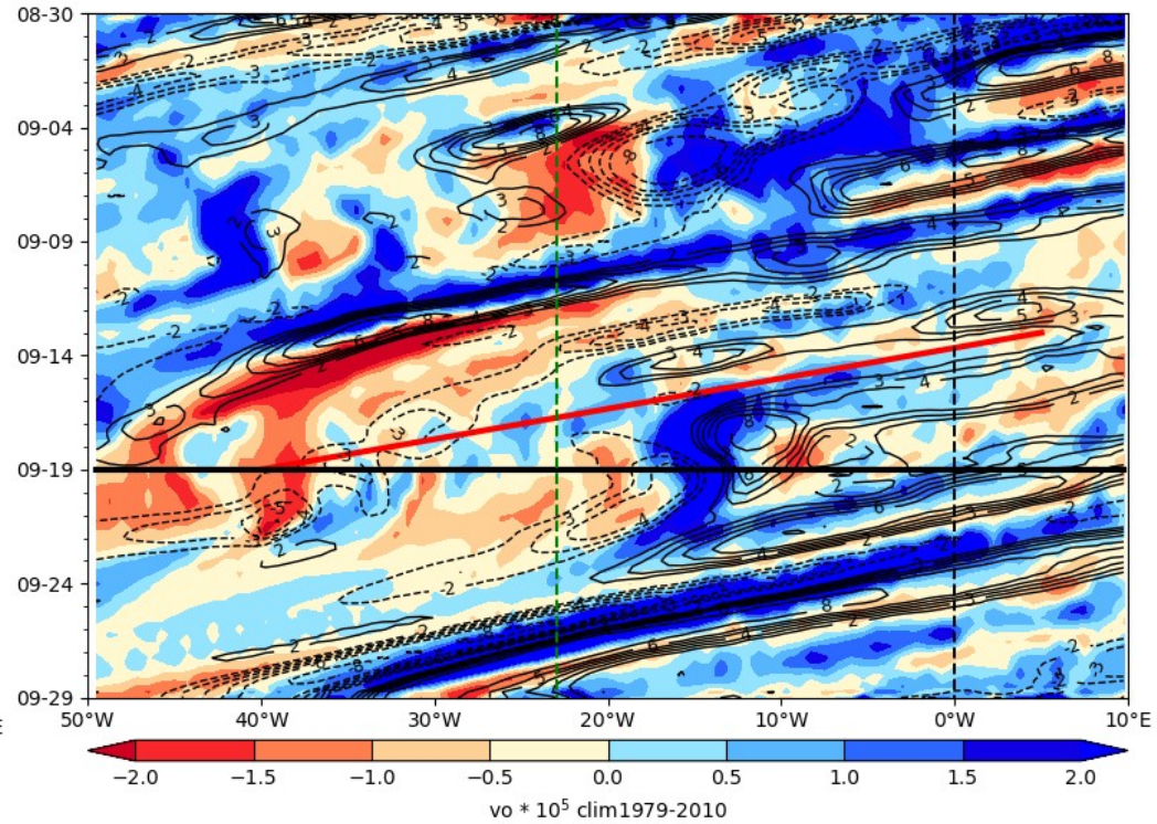
ECMWF Vorticity 850 hPa (color), V-700 hPa 2024-09-19
