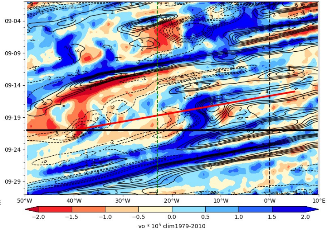
ECMWF Vorticity 850 hPa (color), V-700 hPa 2024-09-21
