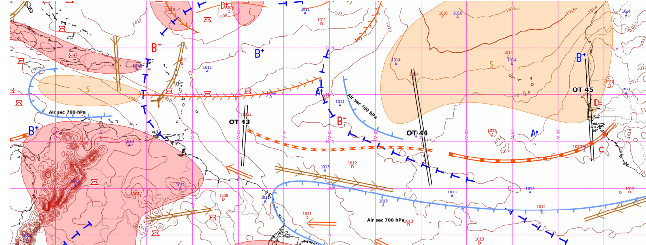
ANASYG du sam. 21/09/2024 - 00 UTC
