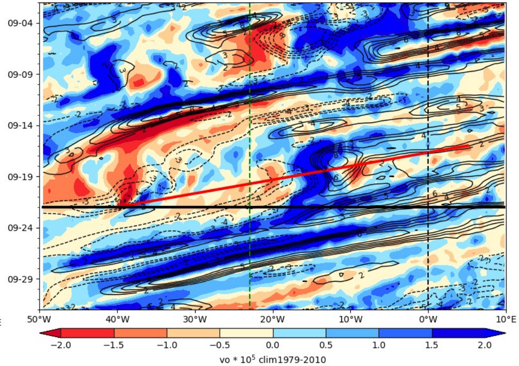
ECMWF Vorticity 850 hPa (color), V-700 hPa 2024-09-22
