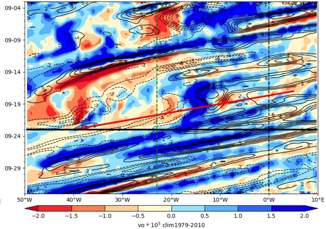
ECMWF Vorticity 850 hPa (color), V-700 hPa 2024-09-23
