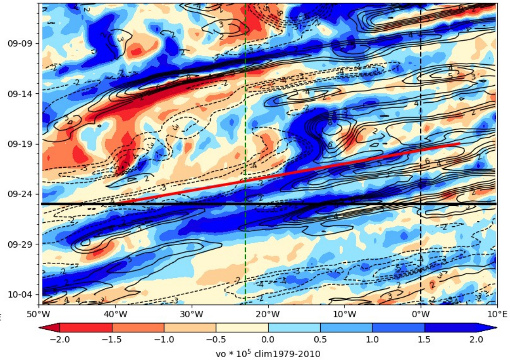
ECMWF Vorticity 850 hPa (color), V-700 hPa 2024-09-25
