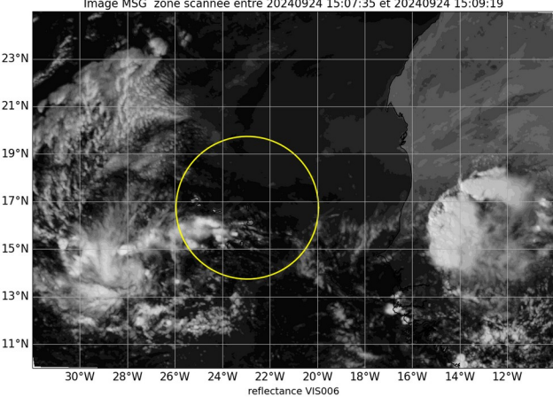
Image MSG zone scannée entre 20240924 15:07:35 et 20240924 15:09:19
