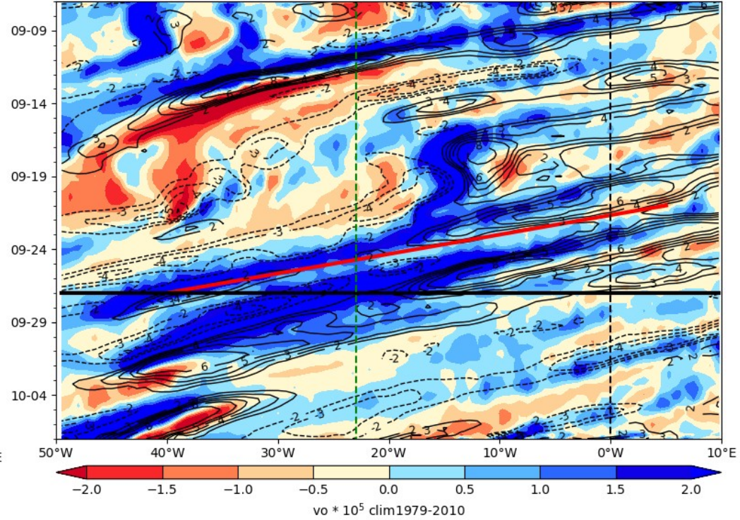
ECMWF Vorticity 850 hPa (color), V-700 hPa 2024-09-27
