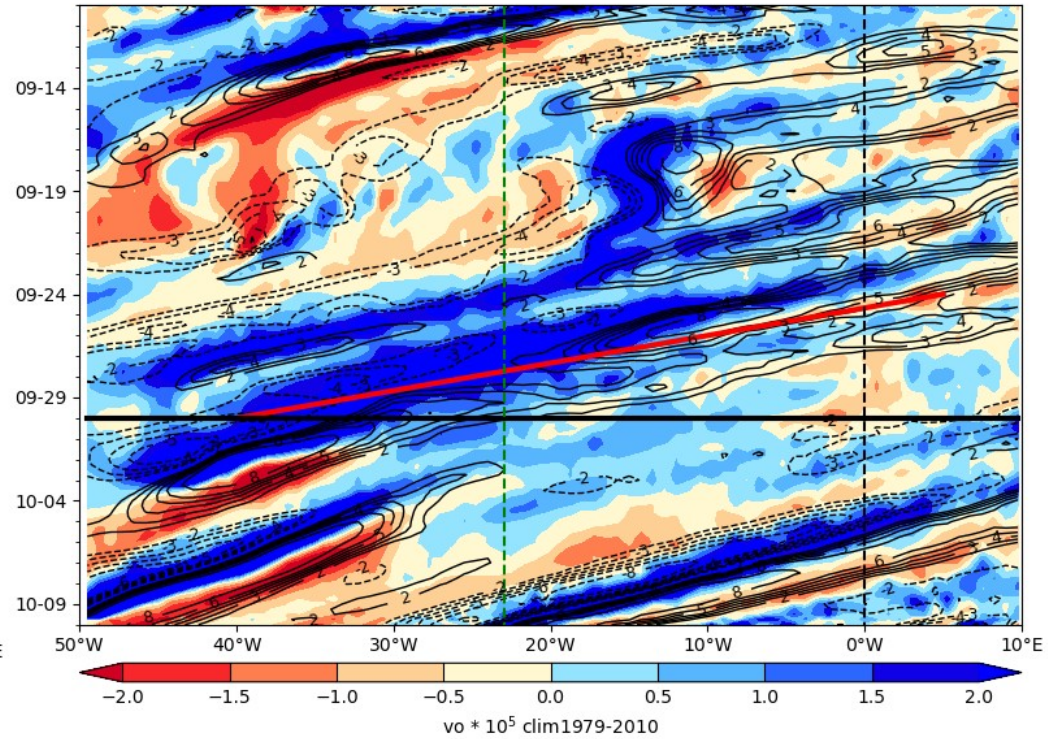
ECMWF Vorticity 850 hPa (color), V-700 hPa 2024-09-30
